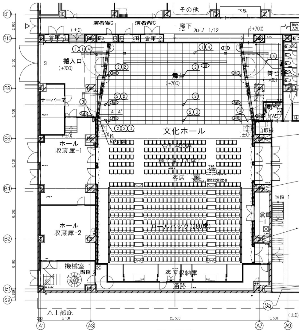
1階平面配置図
