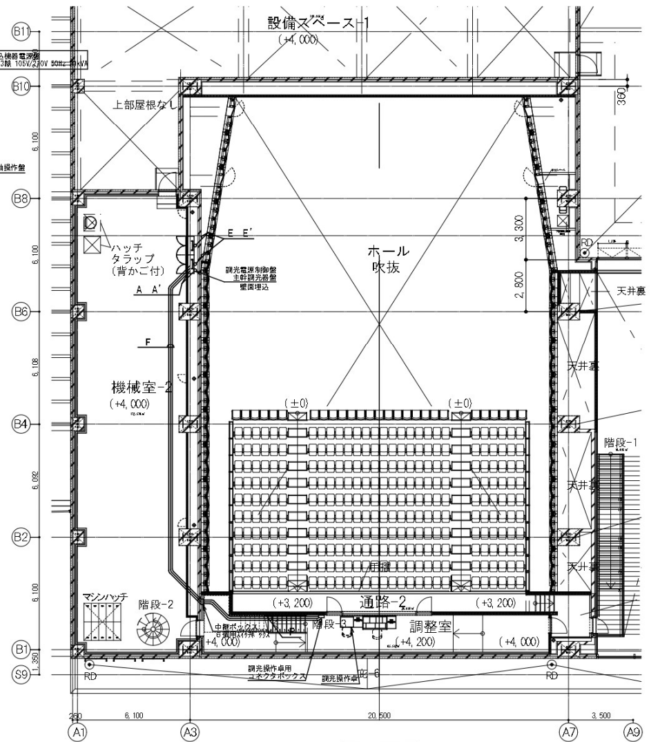
2階平面配置図
