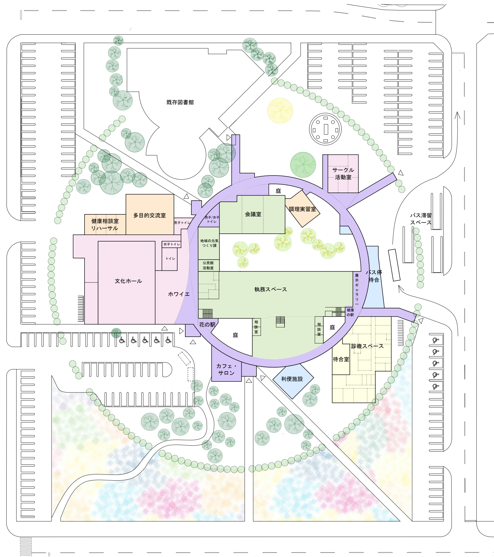
1階平面図 S=1:800
